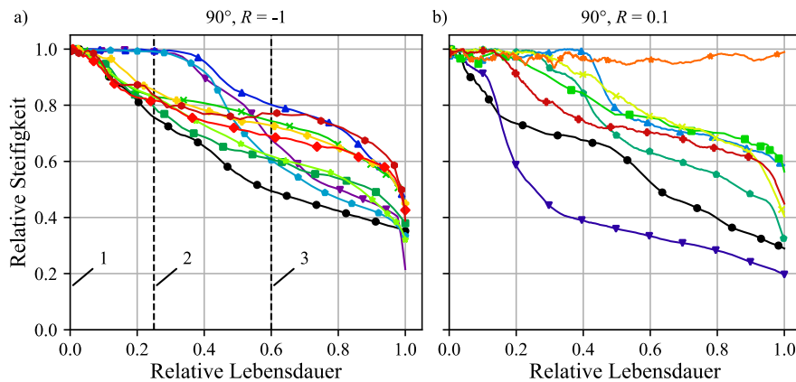
Abbildung 1: Relative Steifigkeitsverläufe quer zur Faser belasteter Faserverbundproben bei unterschiedlichen Lastverhältnissen
