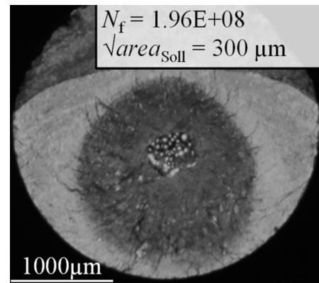
Bruchfläche einer im VHCF-Bereich versagten Probe [1]
